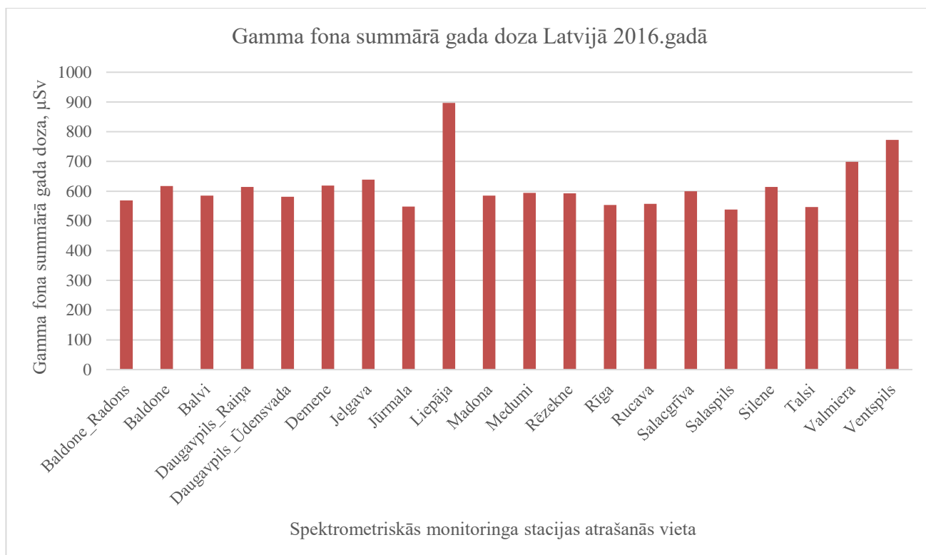
1.att. Summārās gada gamma dozas, 2016. gads
