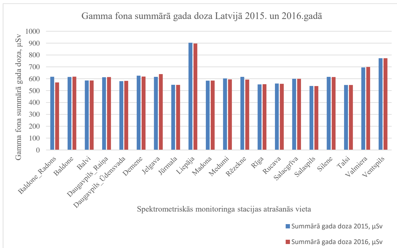
2.att. Summārās gada gamma dozas, 2015.un 2016. gads
